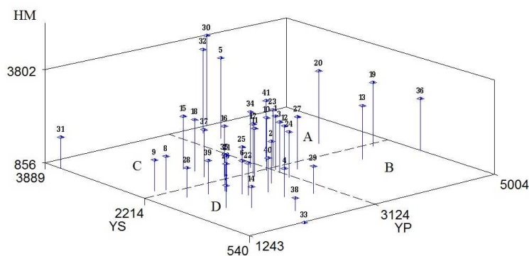
شکل ۱- پراکنش سه بعدی ارقام مورد مطالعه بر اساس شاخص‌های YP (عملکرد در شرایط بدون تنش)، YS (عملکرد در شرایط تنش) و HM (میانگین هارمونیک)
