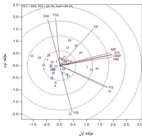
شکل ۲- نمایش بای پلات شاخص‌های تحمل و حساسیت به شوری در ارقام گندم بر اساس اولین و دومین مولفه اصلی. YP عملکرد در شرایط بدون تنش، YS عملکرد در شرایط تنش، SSI شاخص حساسیت به تنش، TOL شاخص تحمل، MP میانگین بهره‌وری، GMP میانگین هندسی بهره‌وری، STI شاخص تحمل به تنش، HM میانگین هارمونیک، YI شاخص عملکرد، YSI شاخص پایداری عملکرد.
