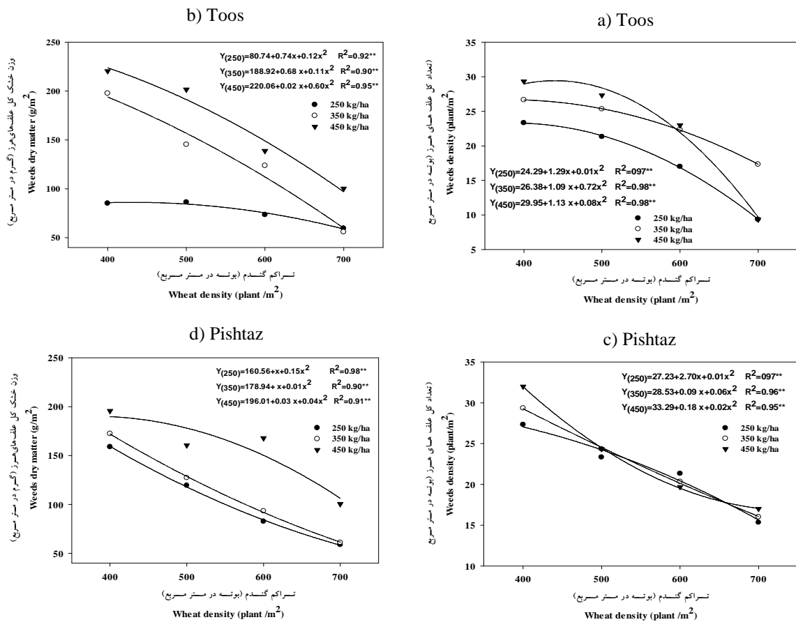
شکل ۶- تاثیر کود اوره و تراکم بوته گندم بر فراوانی و وزن خشک کل علف‌های هرز. a و b) رقم توس، c و d) رقم پیشتاز. Figure 6. Effect of urea fertilizer and wheat density on the frequency and dry weight of total weeds density. a and b) Toos, c and d) Pishtaz.
