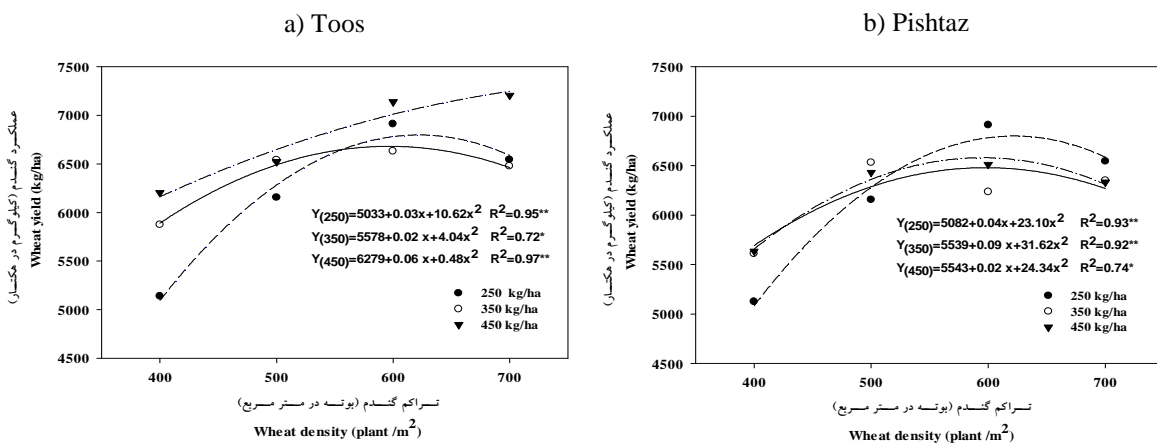
شکل ۷- تاثیر کود اوره و تراکم بوته بر عملکرد دانه دو رقم گندم. a) رقم توس، b) رقم پیشتاز. Figure 7. Effect of urea fertilizer and wheat density on grain yield of two wheat varieties. a) Toos, b) Pishtaz.
