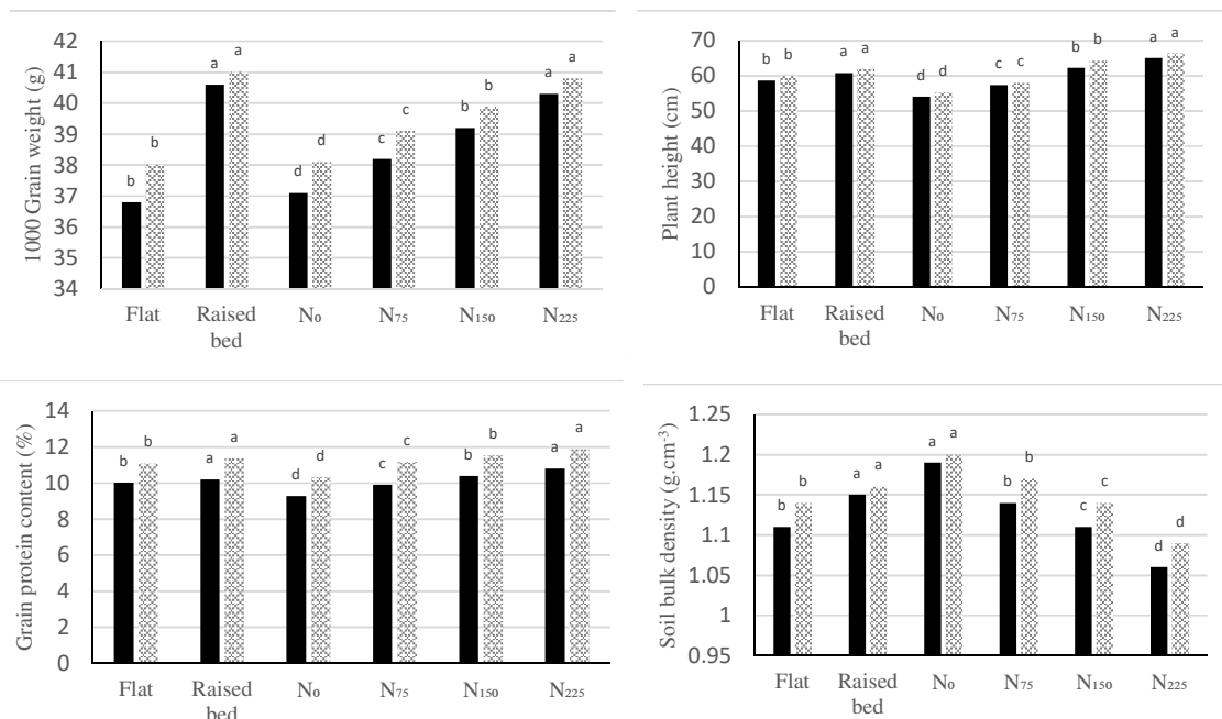
شکل ۱- مقایسه میانگین صفات گیاهی گندم و وزن مخصوص خاک در تیمارهای روش کاشت و کود نیتروژن (سال اول ■ سال دوم) Figure 1. Mean comparison of wheat plant traits and soil bulk density in planting method and nitrogen fertilizer treatments (first year ■ second year)
